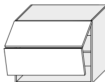
W8B/90 - AV 900/720/325
