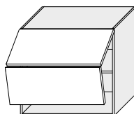
W8B/80 - AV 800/720/325
