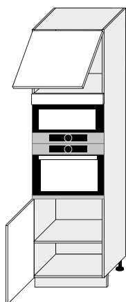
D14/RU/60/207 600/2070/565
