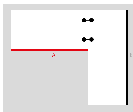
Typ spoje pracovní desky L1 Rozměry vždy uvádějte dle nákresu v cm
