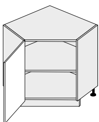
D12R/90 840/820/840
