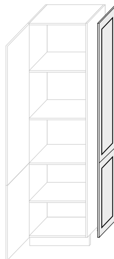
FBW 07 590x1970x19
